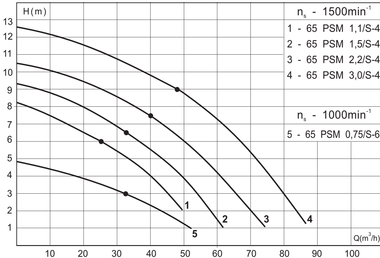
Rys.1. CHARAKTERYSTYKA HYDRAULICZNA POMP TYPU 65 PSM.../S-4 i S-6
