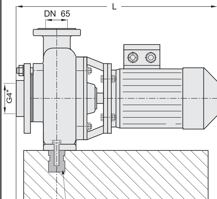
Rys.4. Wymiary gabarytowe i instalacyjne pomp 65 PSM
