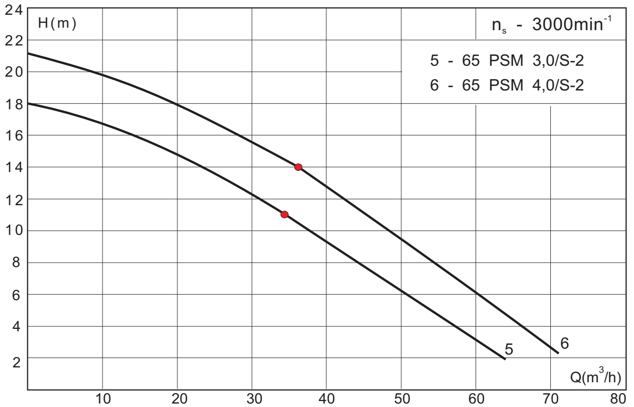
Rys.2. CHARAKTERYSTYKA HYDRAULICZNA POMP TYPU 65 PSM.../S-2
