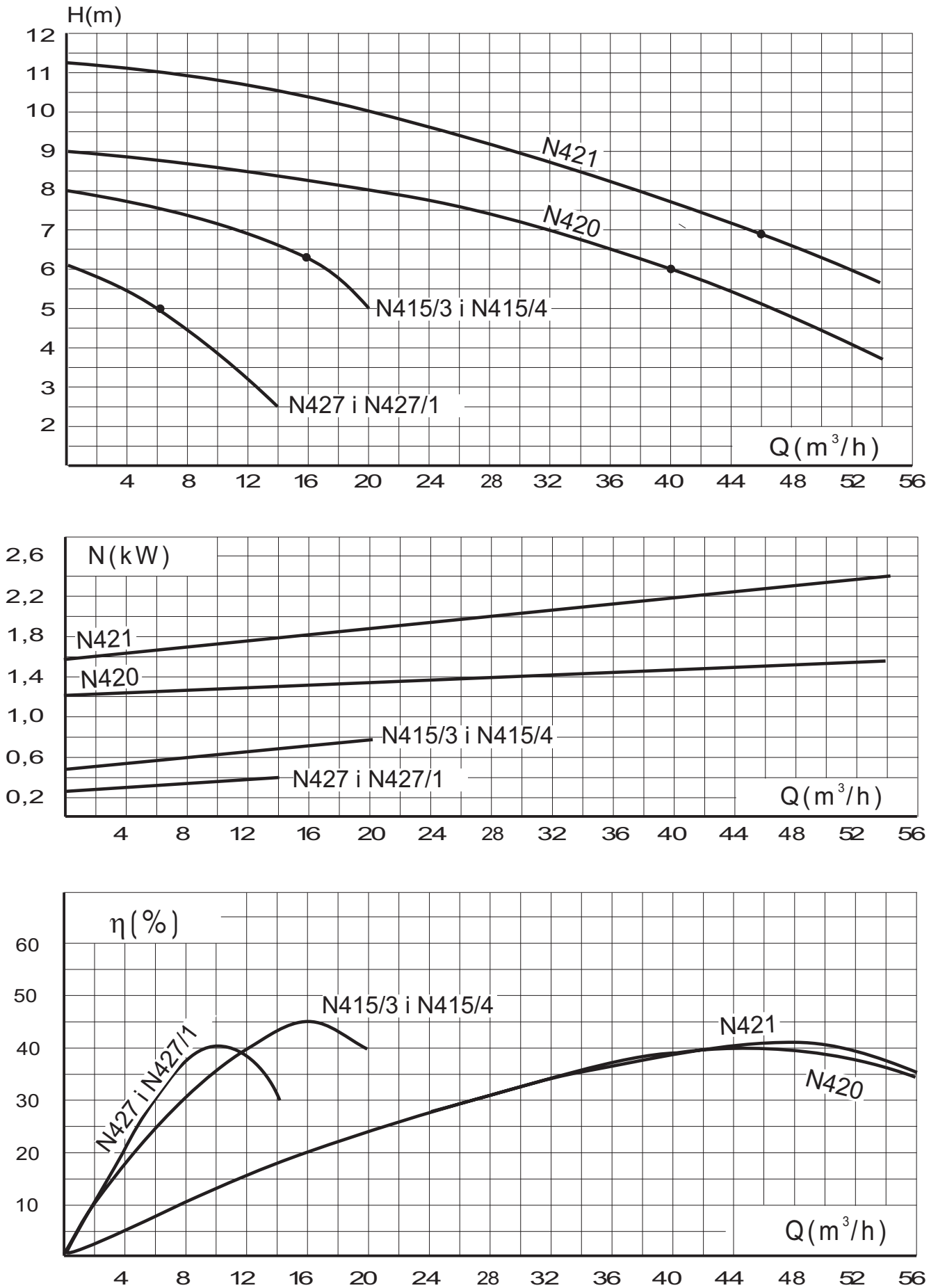
Rys 1. Charakterystyka hydrauliczna pomp typu: N427, N427/1, N415/3, N415/4, N420 i N421
